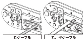
丸ケーブル
