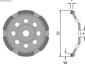
寸法図 CSA4 シングル
