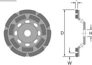
寸法図 CDA4 ダブル
