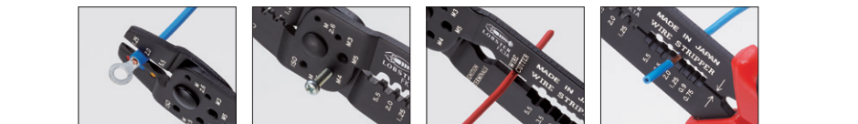
絶縁端子圧着歯口 (1.25、2、5.5mm) ボルトカッター (適用サイズM2.6～M5) ワイヤーカッター ワイヤーストリッパー (適用サイズ0.75～5.5mm)
