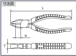
J200PC
