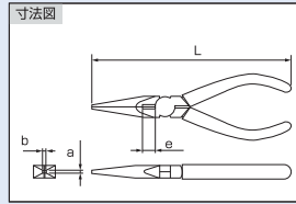
ハネ部 (J100R/J115R/J150RS)
