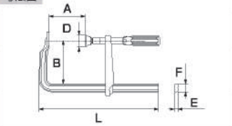
寸法図
