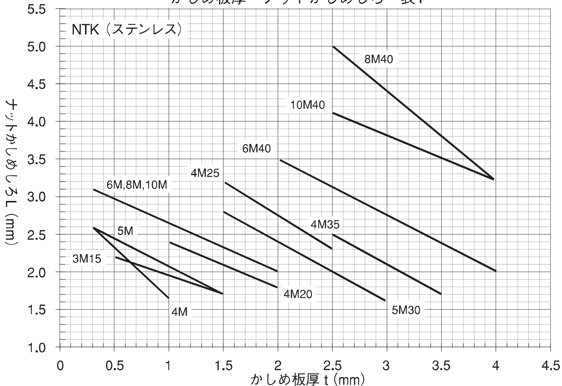
かしめ板厚－ナットかしめしろ 表1
