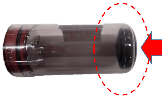
タンクの底部（矢印部）にクラック
